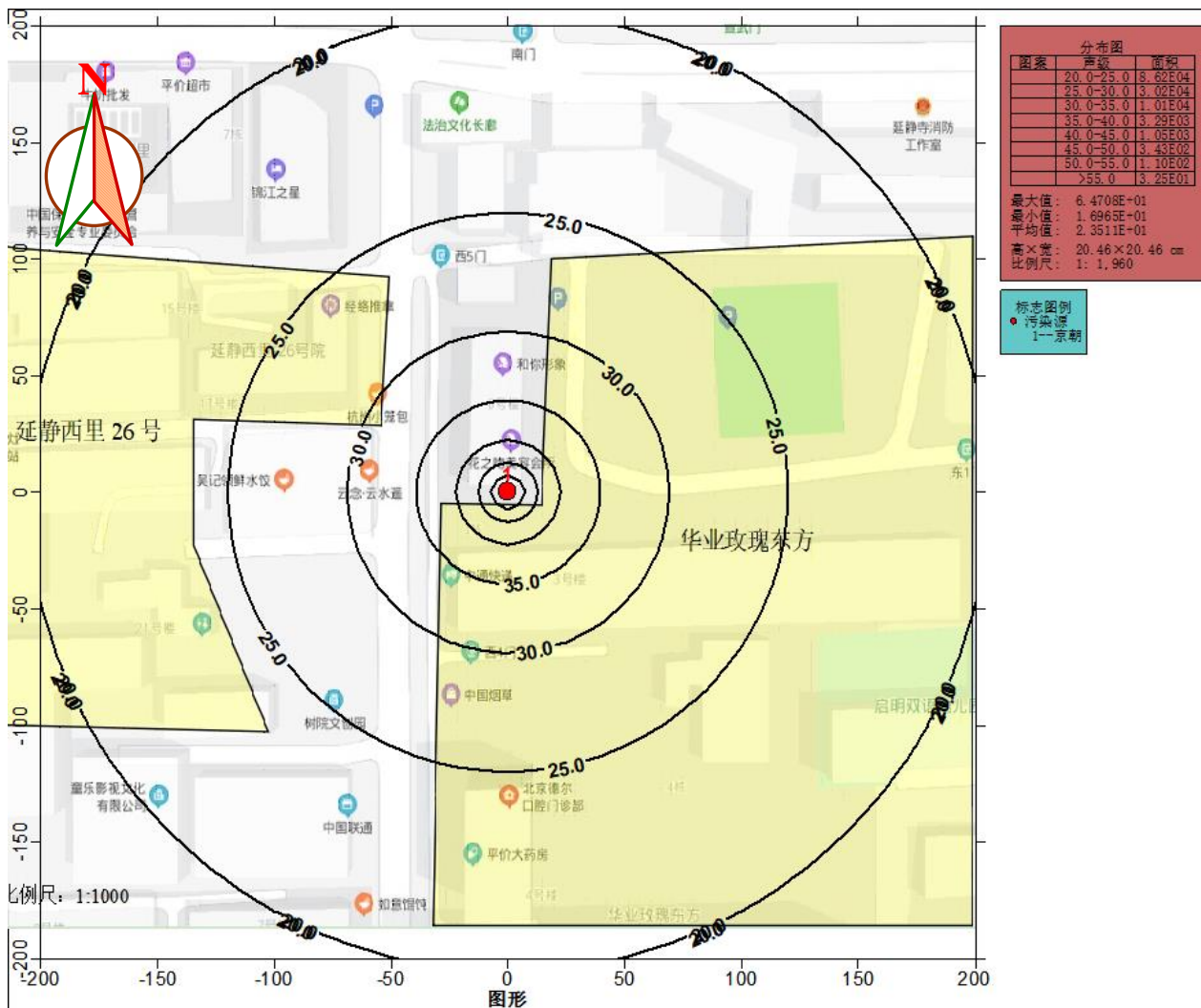
图 7 等声级线图
