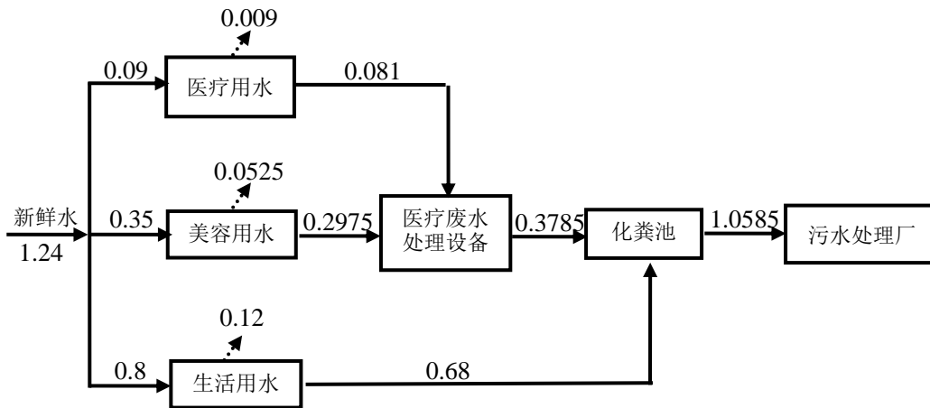
图 1 给排水平衡图 m 3 /d
