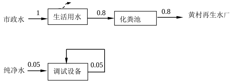
图1 建设项目水平衡图 单位： \text{m}^3/\text{d} “↗”消耗量
