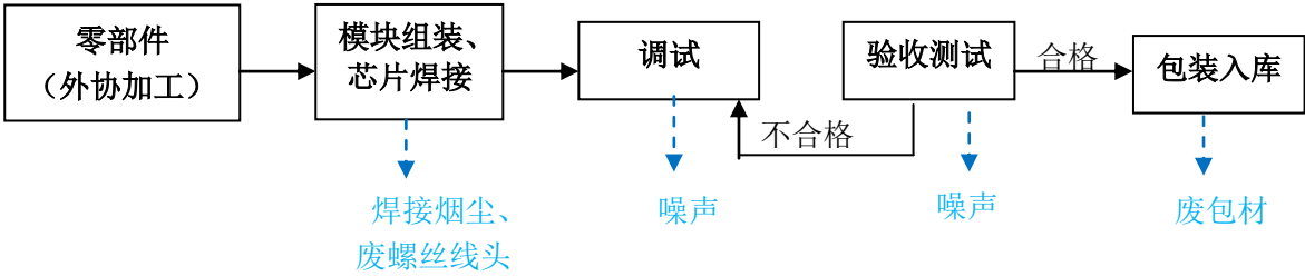
图 2 泵浦光源工艺流程图
