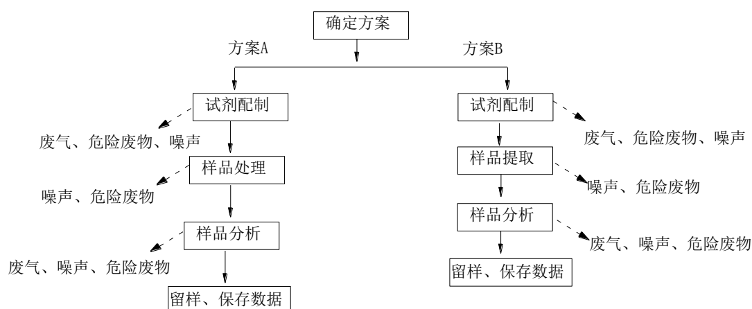
图2 项目工艺流程及产污节点图
