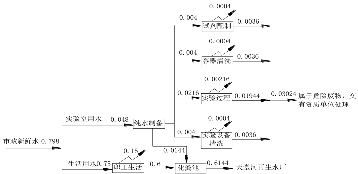
图 1 建设项目水平衡图 单位: m 3 /d “ ”消耗量
