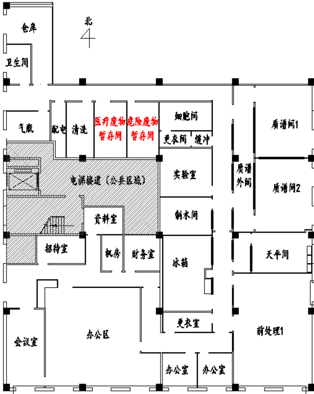
附图 3 项目平面布置示意图
