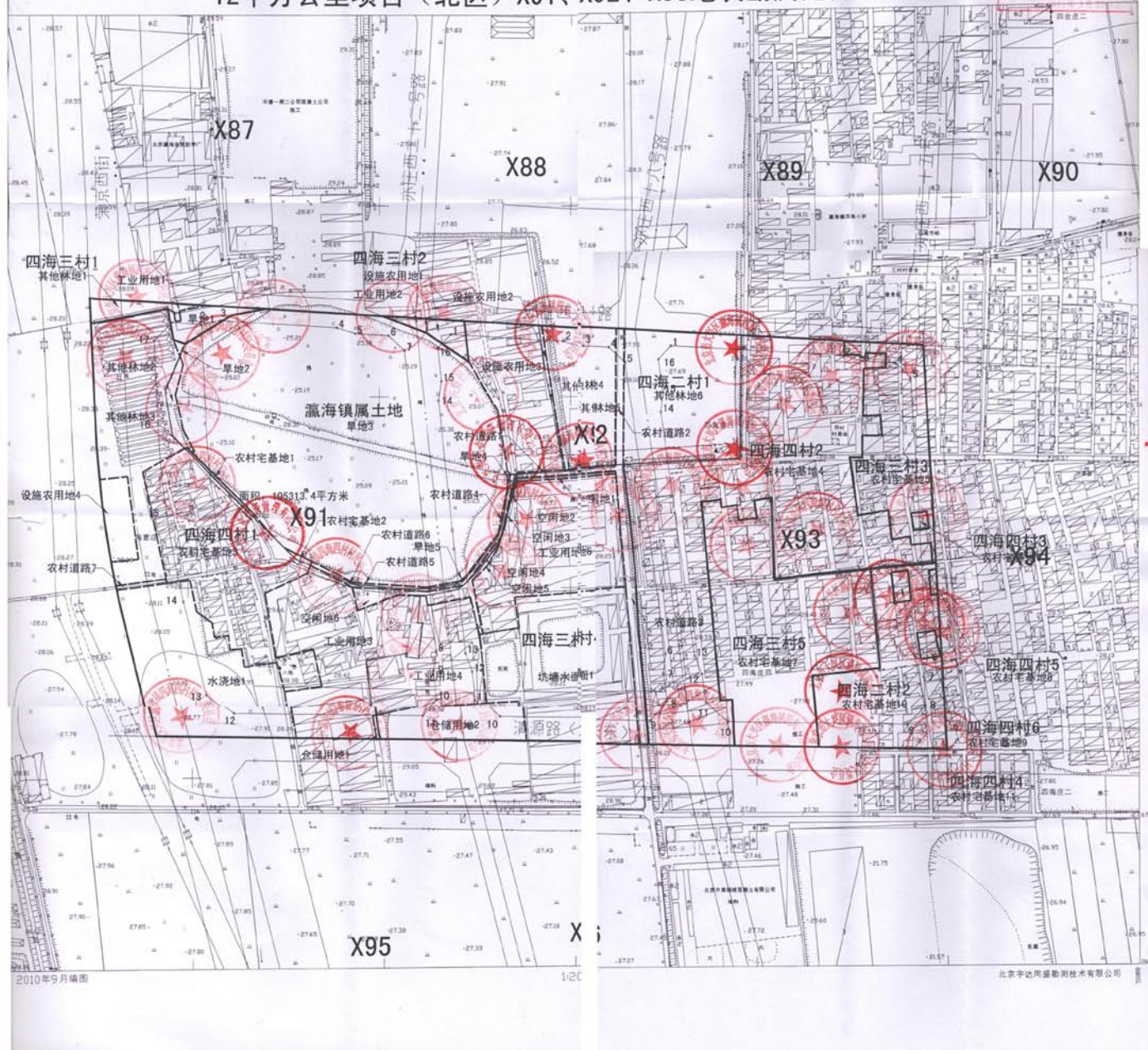
12平方公里项目（北区）X91、X92、X93地块勘测定界成果图
