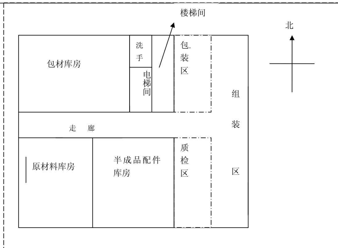
图 3 项目生产车间平面布置图
