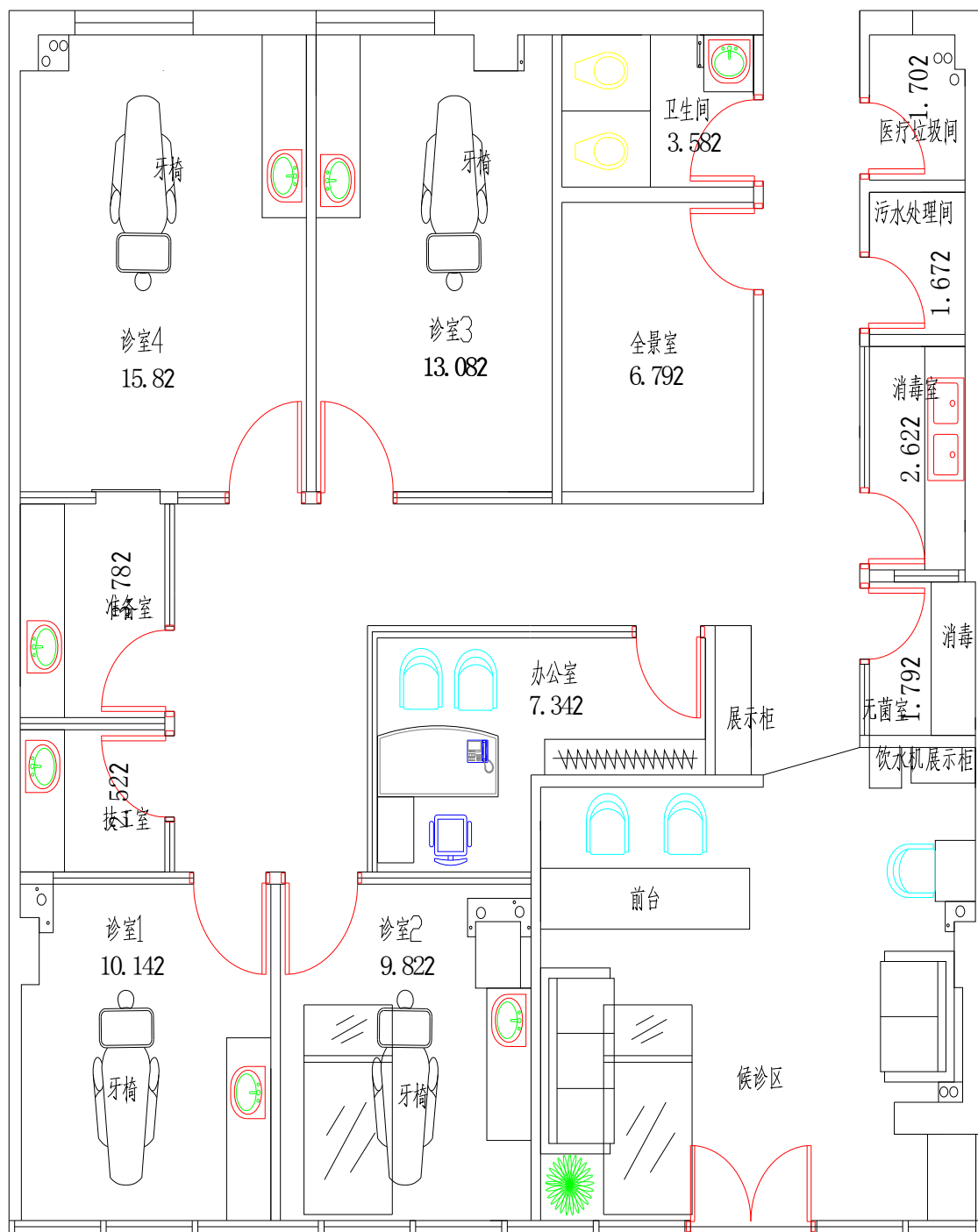
图3 项目平面布置图
