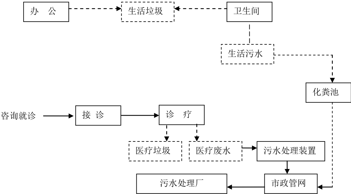
建设项目工艺流程及产污环节示意图
