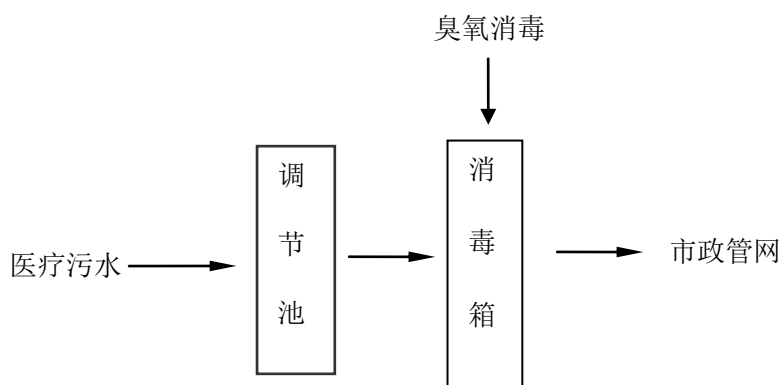
项目医疗废水处理工艺流程示意图
