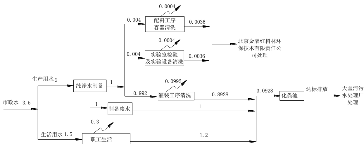
图 1 建设项目生产期间水量平衡图 单位: m³/d
