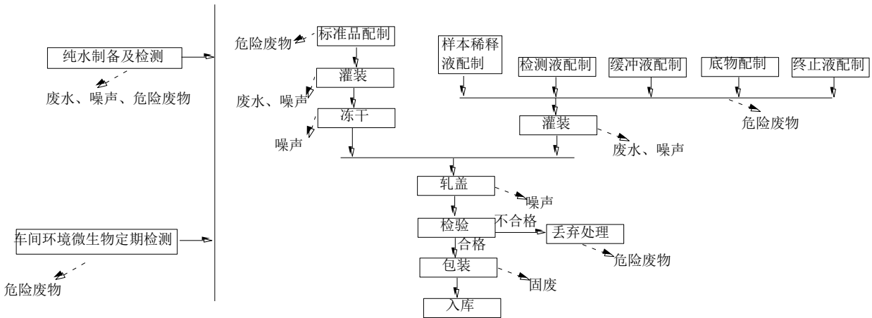
图 3 人体甘胆酸检测试剂盒工艺流程及其产污节点图
