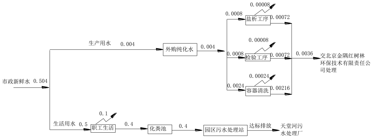
图1 建设项目生产期间水量平衡图 单位: m³/d “N”消耗量
