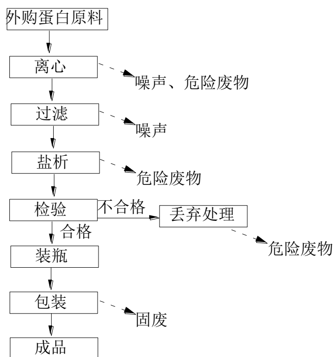
图 2 蛋白材料生产工艺流程及其产污节点图
