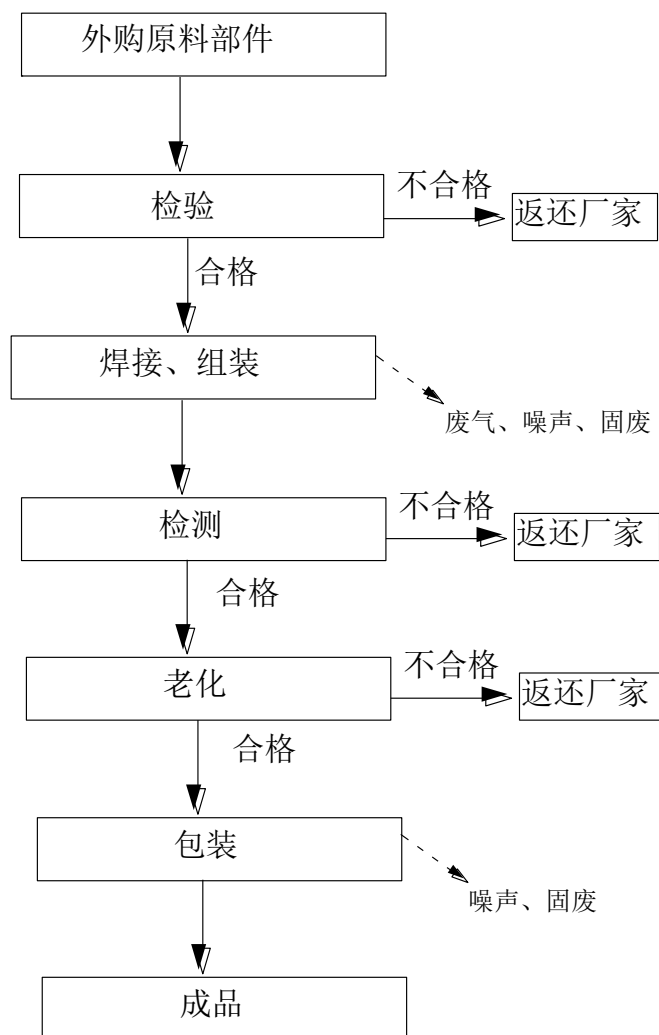
图2 项目工艺流程及其产污节点图
