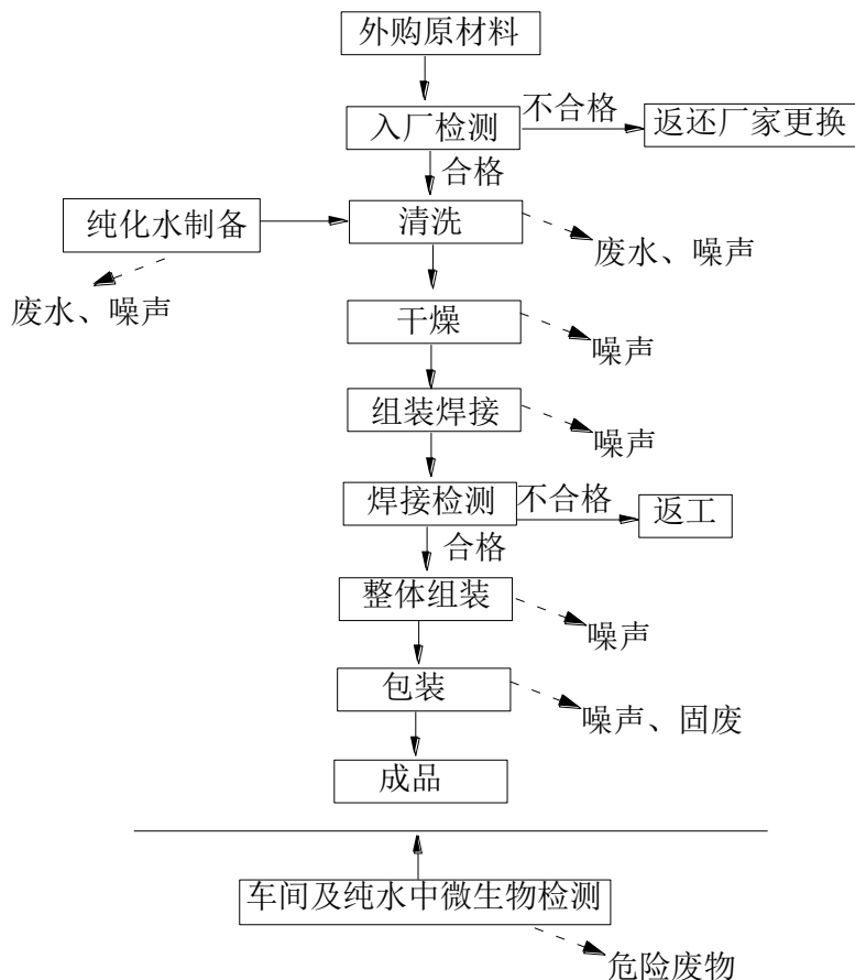
图 2 外科手术器械生产工艺流程及其产污节点图
