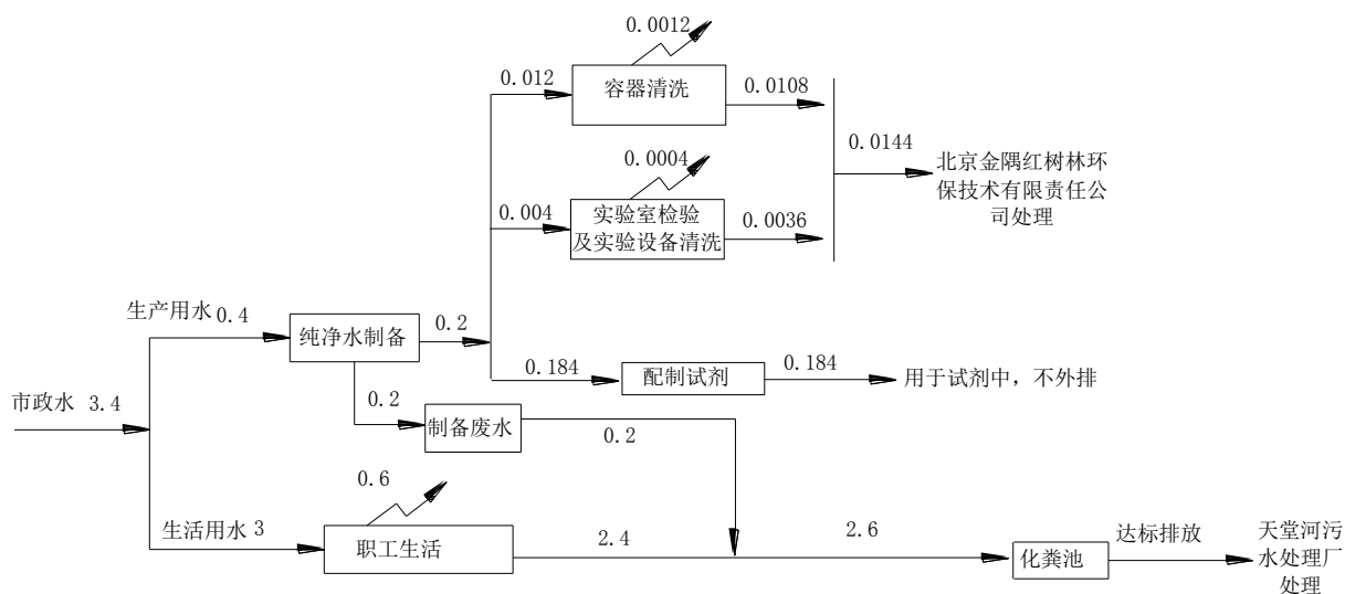
图 1 建设项目生产期间水量平衡图 单位: \text{m}^3/\text{d} “” 消耗量
