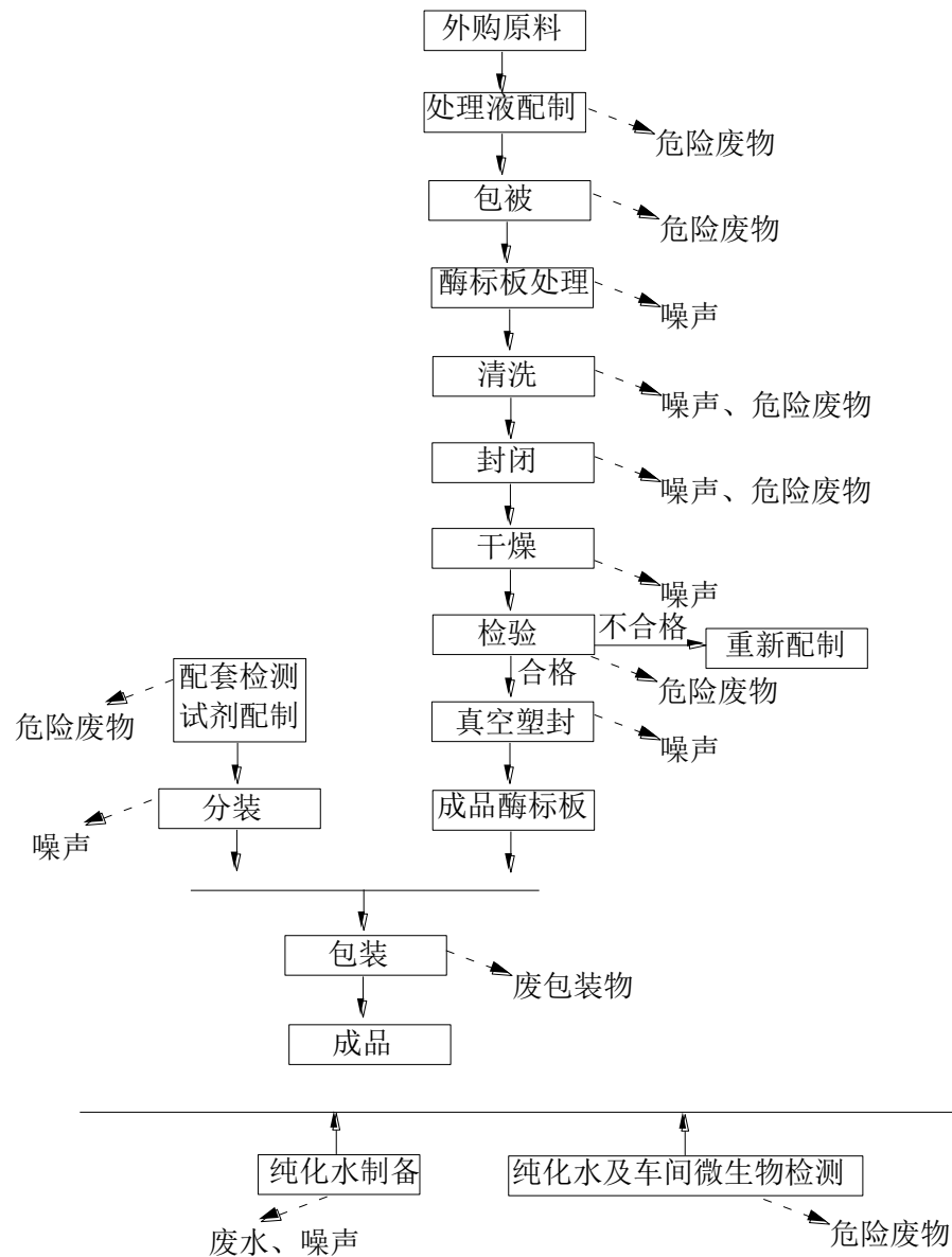
图 3 酶联免疫类产品工艺流程及其产污节点图
