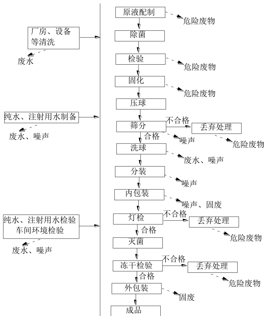
图 2 海藻酸钠微球血管栓塞剂生产项目工艺流程及其产污节点图
