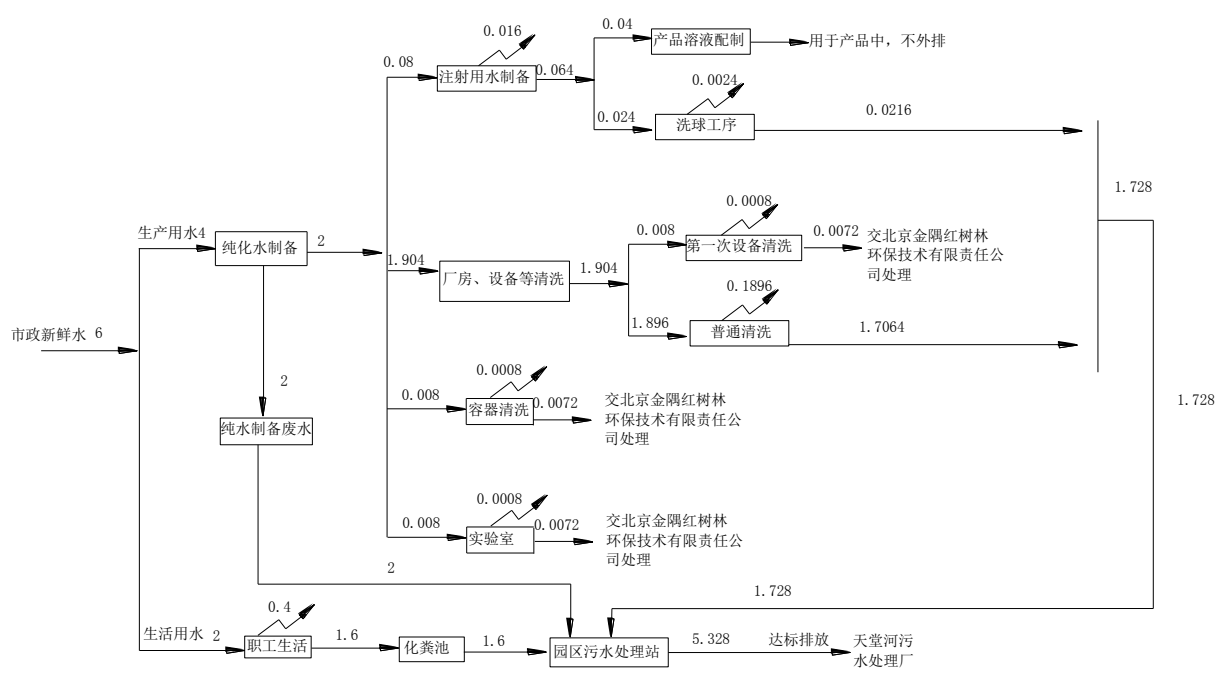
图 1 建设项目生产期间水量平衡图 单位：m³/d “N” 消耗量
