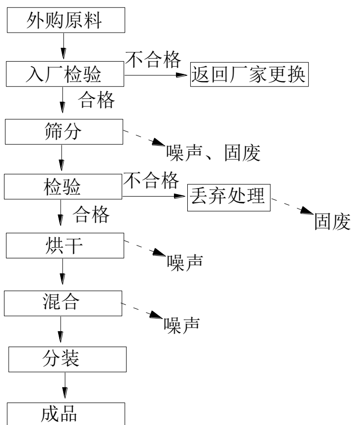
图 1 齿科烤瓷合金粉末工艺流程及其产污节点图
