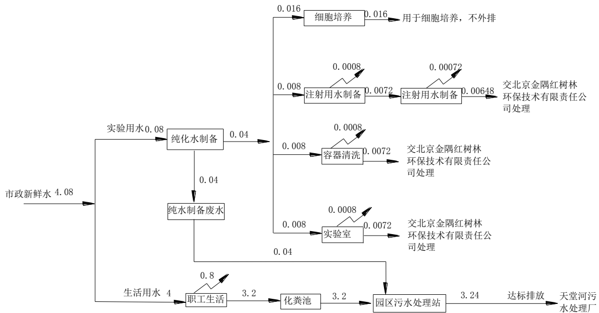
图 1 建设项目运营期间水量平衡图 单位: \text{m}^3/\text{d} “消耗量”
