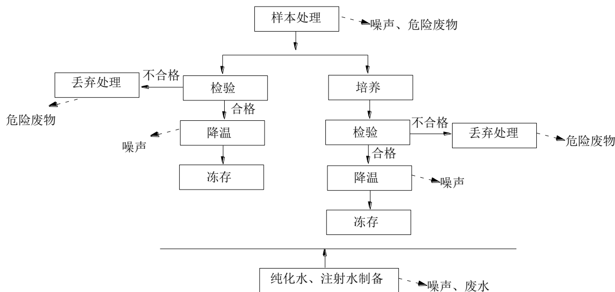
图 2 研发实验工艺流程及其产污节点图
