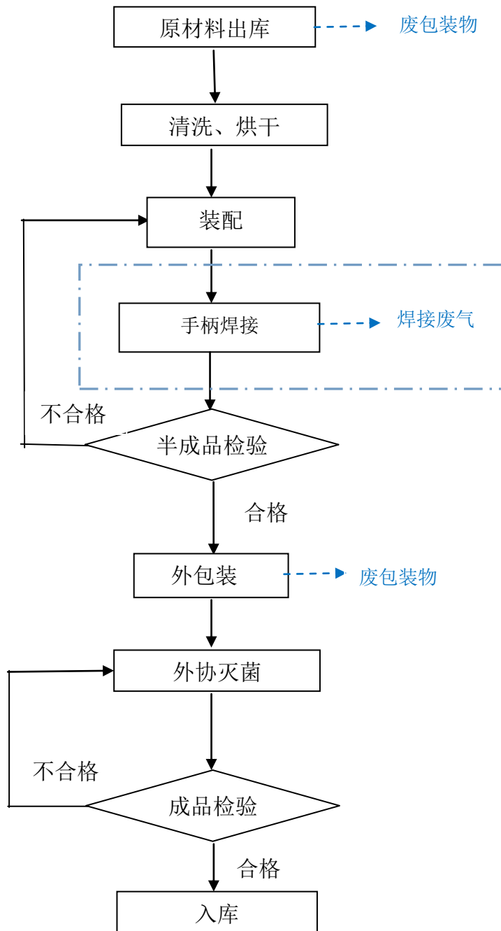
图 2-2 耗材类产品工艺流程及其产污节点图
