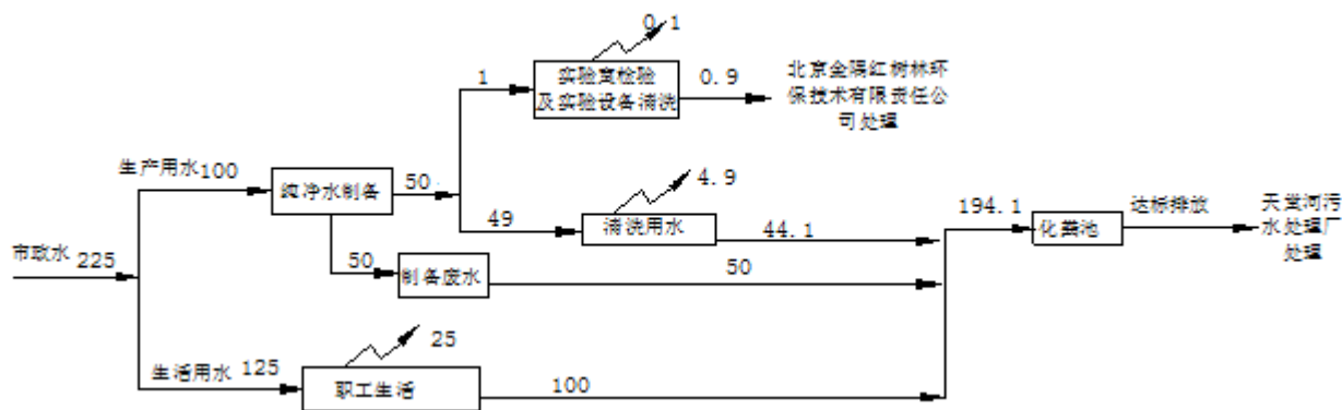
图 3-4 项目给排水平衡图 单位： \text{m}^3/\text{a}
