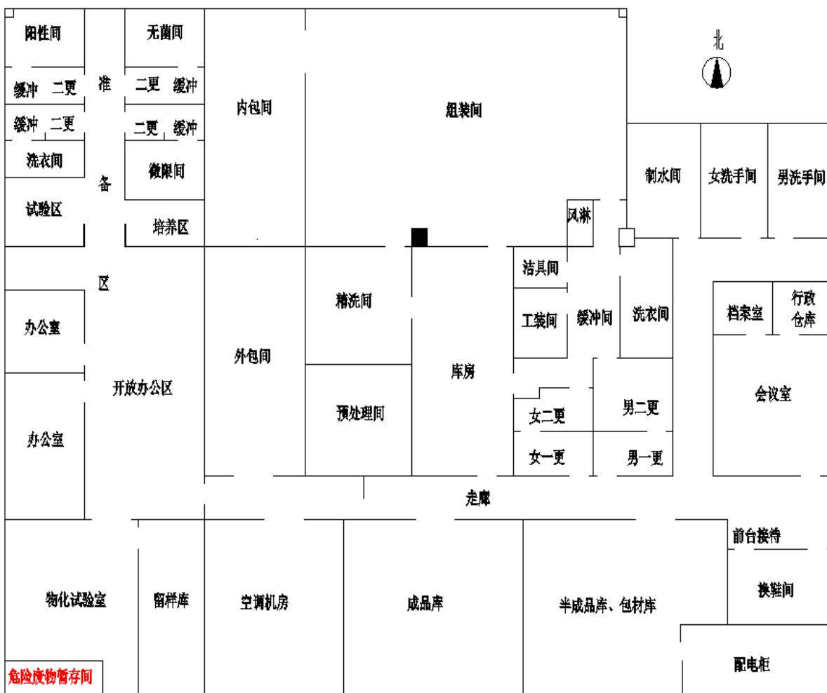
图 3-3 本项目平面布置图
