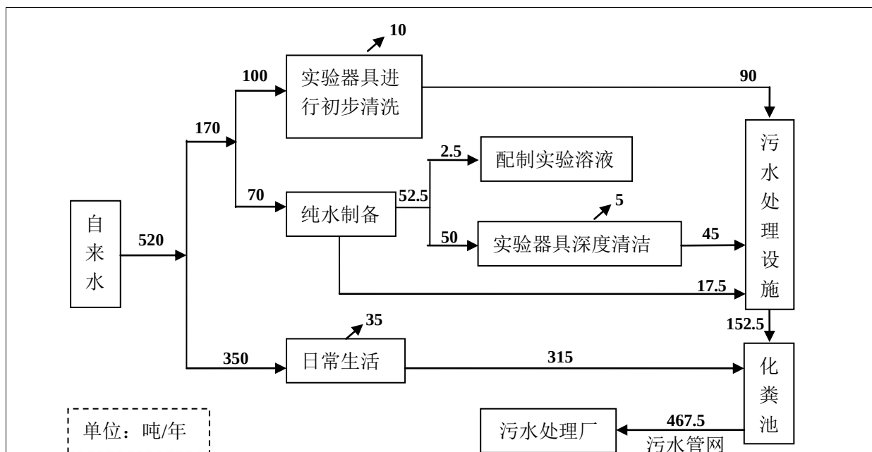
图 6 水量平衡图
