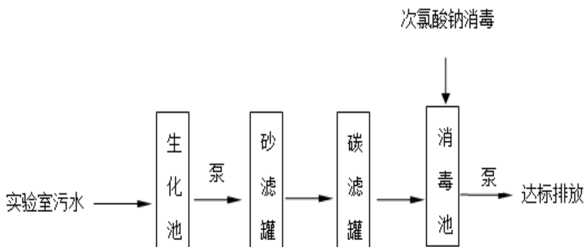
图 7 废水处理工艺流程
