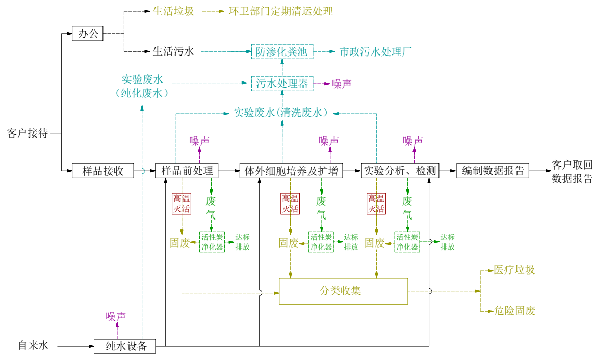
图 4 运营期间工艺流程及产污环节示意图
