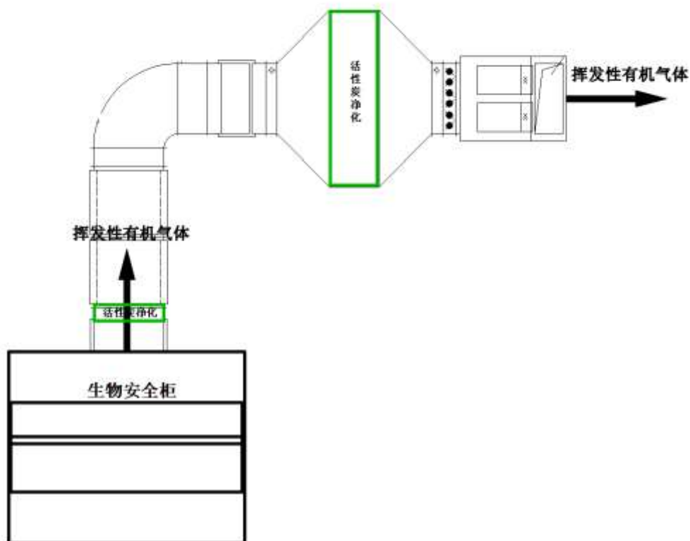
图 5 废气经过活性炭净化处理示意图
