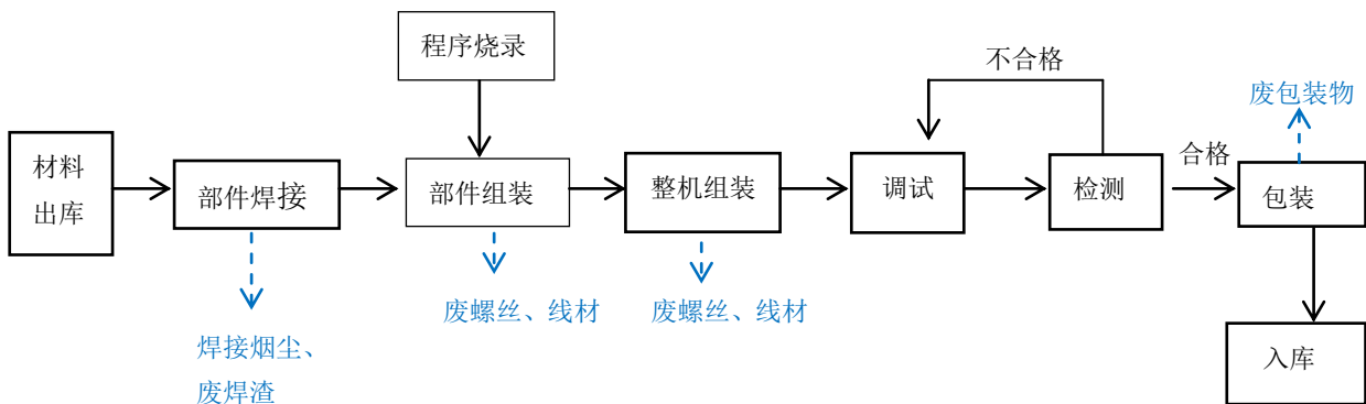
图 3 工艺流程及产污节点图
