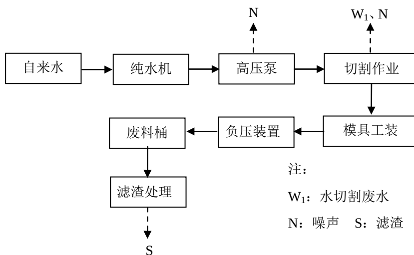
图 4 水切割工艺流程图
