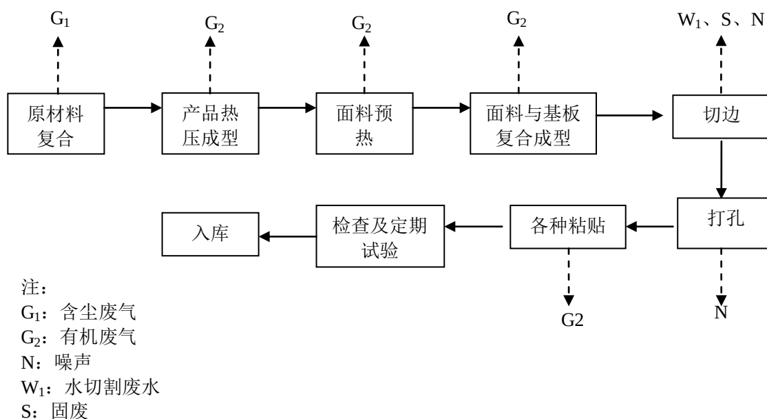
图 2 湿法顶棚工艺流程图
