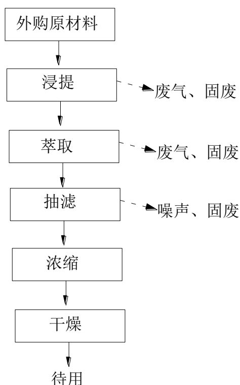
图 2 提取工艺流程及产污节点图
