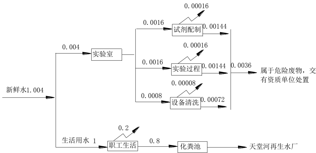
图1 建设项目水平衡图 单位：m 3 /d “⚡” 消耗量
