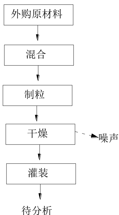
图 4 颗粒剂工艺流程及产污节点图
