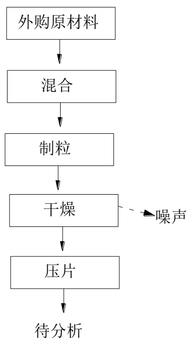
图 3 片剂工艺流程及产污节点图
